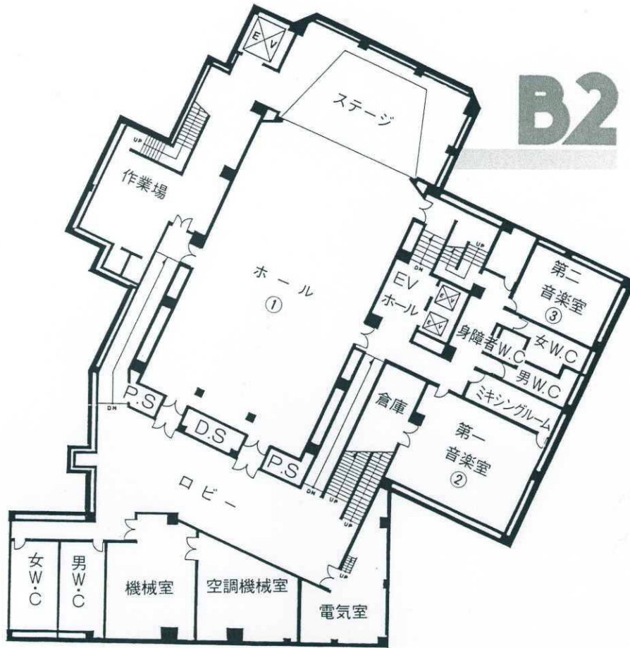
平面図
